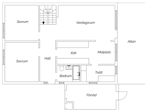
Entréplan
