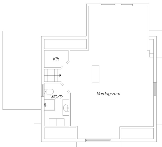
Övre plan
