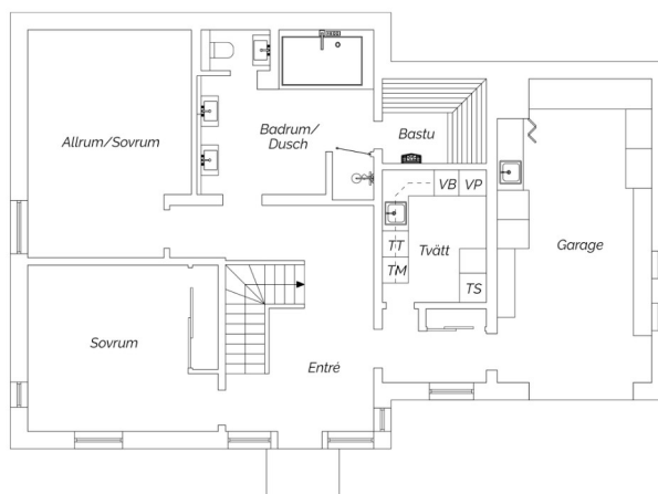
Entréplan
