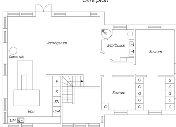
Övre plan
