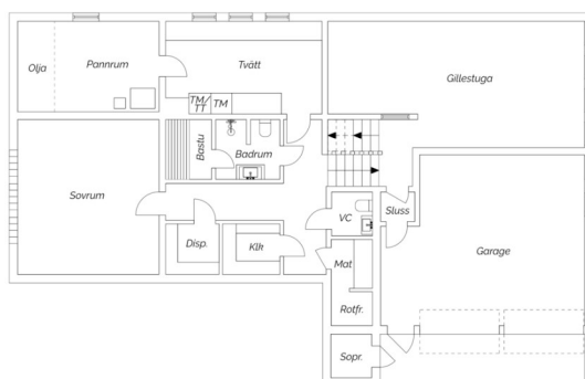
Källarplan
