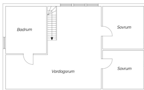
Ovanvåning
